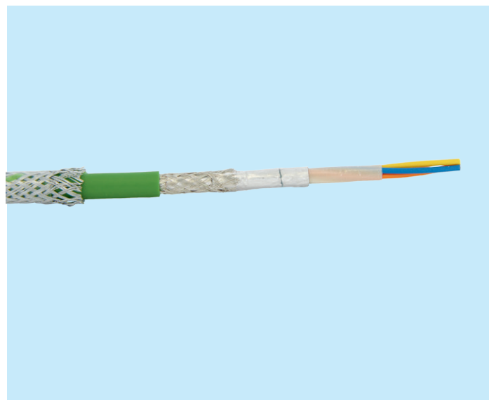
PROFINET-Cable Cat5 Typ A, solid +FE
