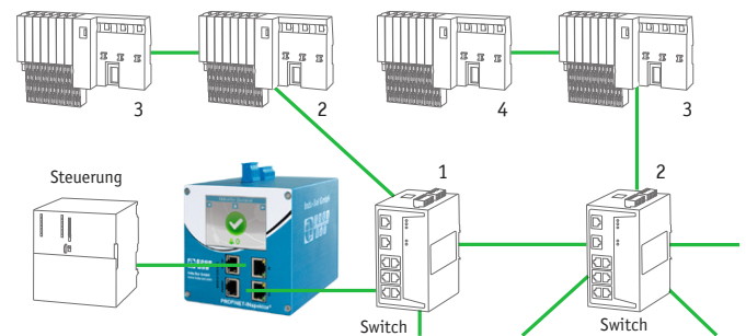
PROFINET-INspektor® NT „Its position in network“
