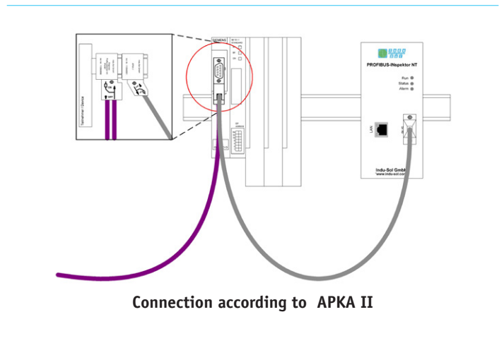
PROFIBUS-INspektor® NT
